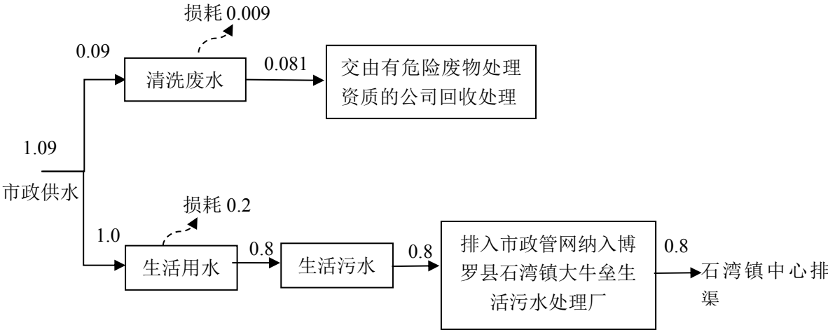
图 2-1 项目水平衡图 (m³/d)
