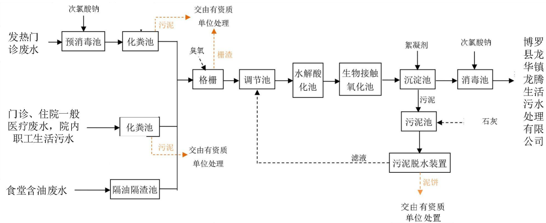
图 4-1 项目拟采用废水处理工艺流程图
