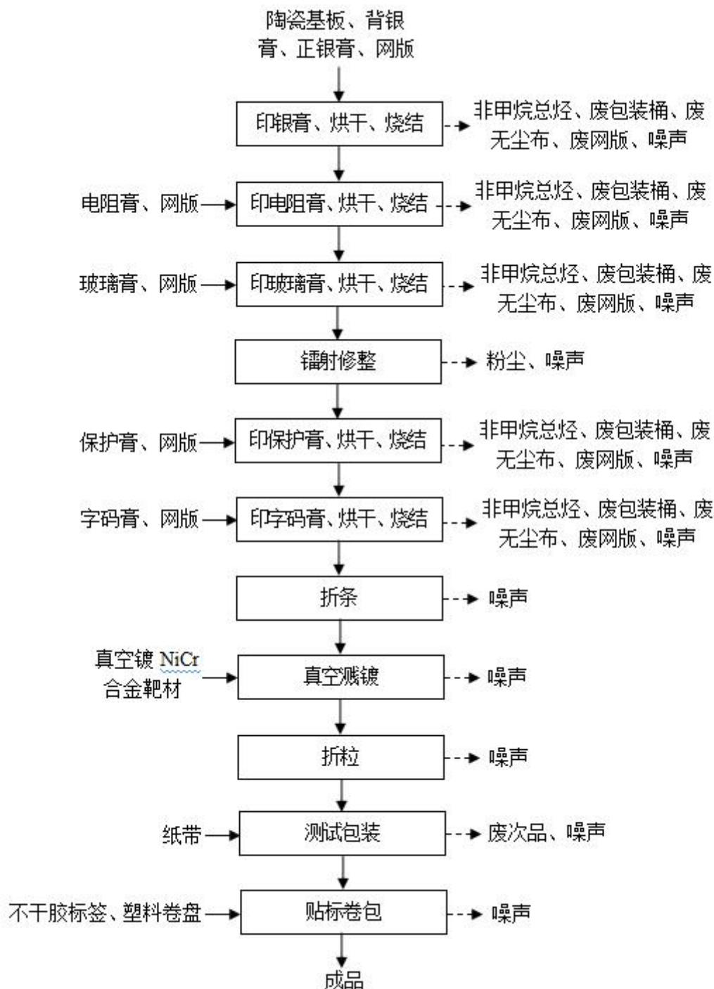
图 2-2 项目生产工艺流程及产污环节图
