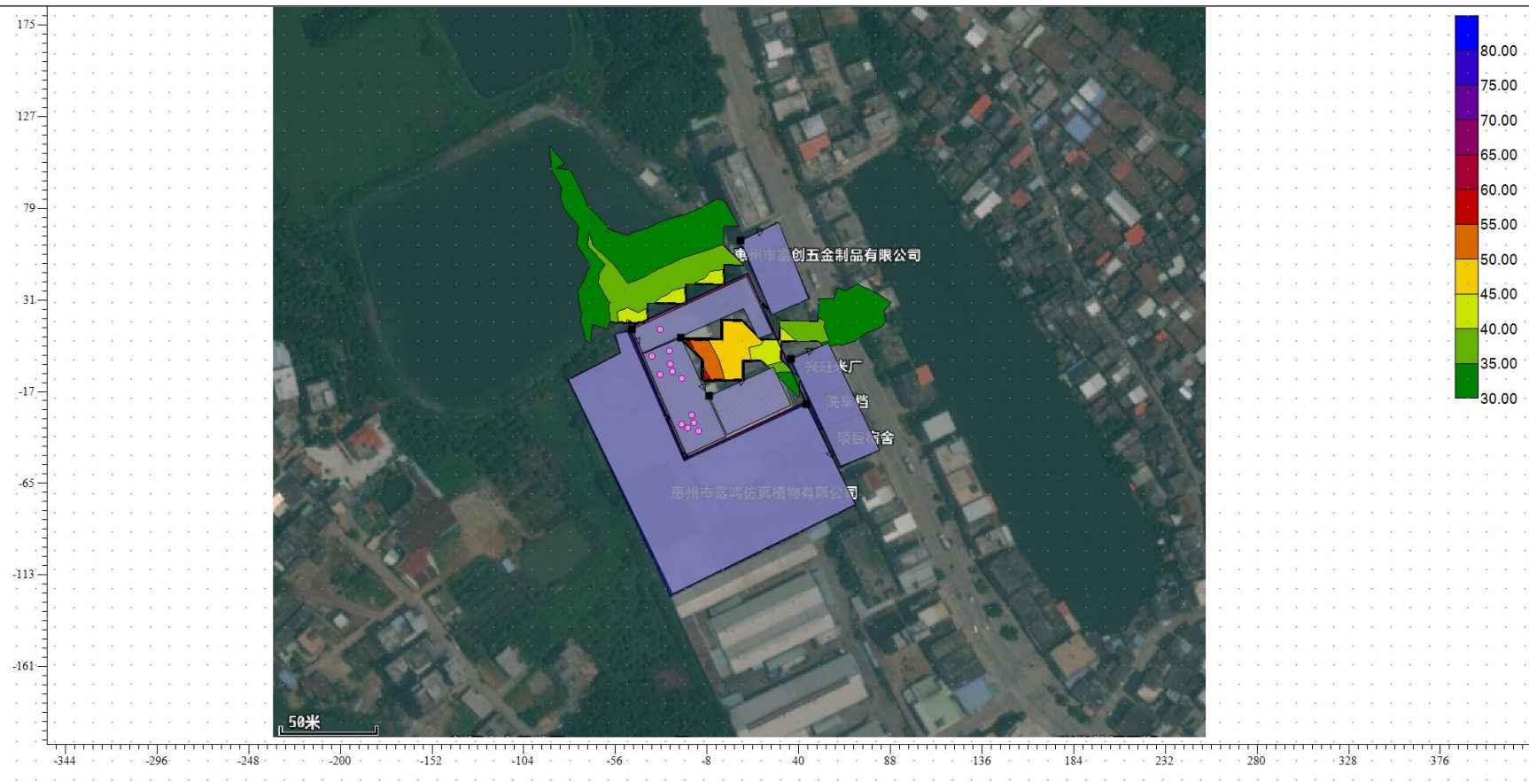
图 4-2 噪声预测图
