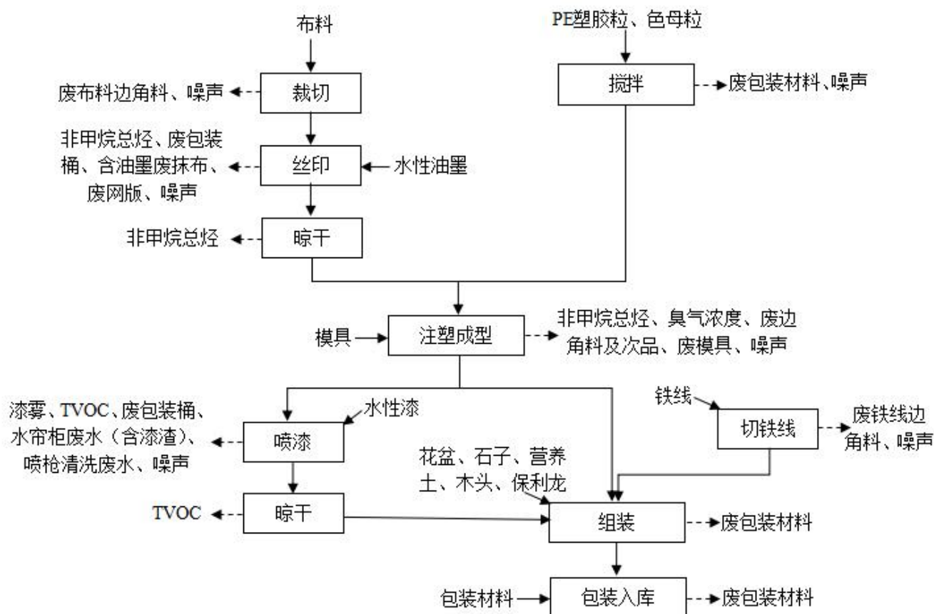
图 2-2 项目工艺流程及产污环节图
