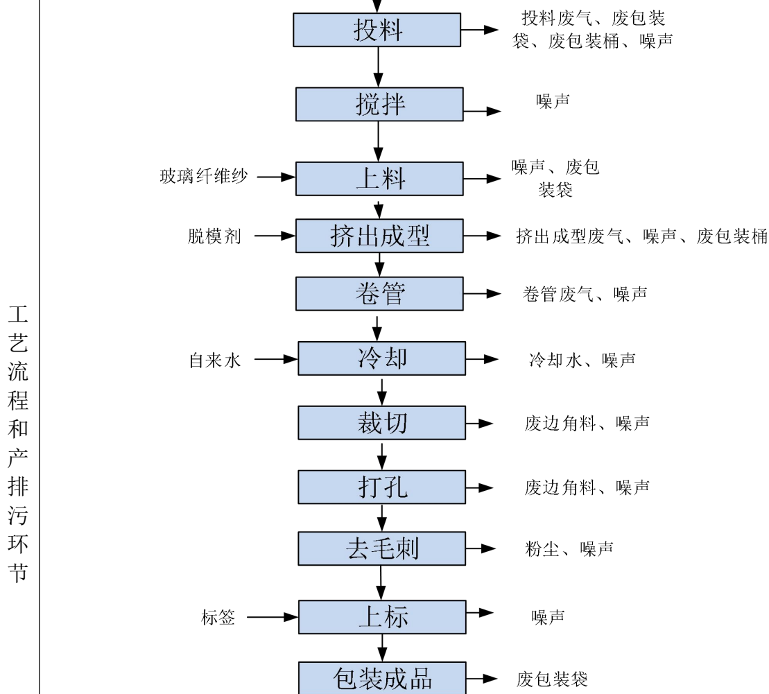
图2-2 项目玻璃纤维管和玻璃纤维杆生产工艺流程图
