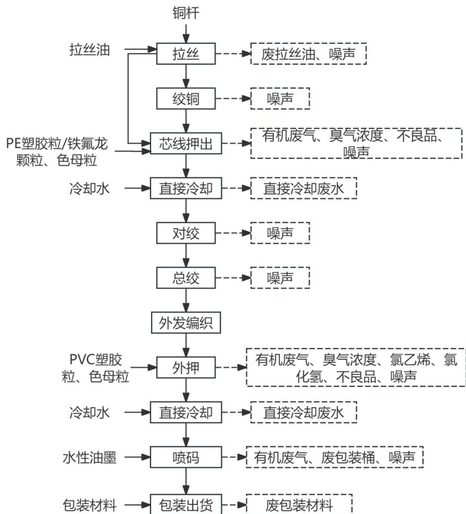
图2-2 网线生产工艺及产污流程图
