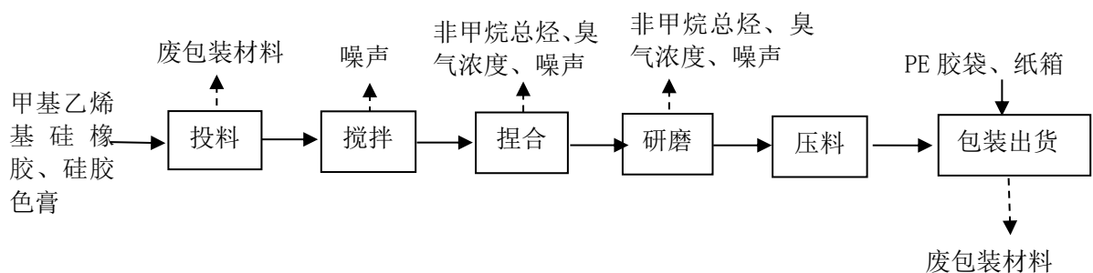
图 2-2 项目硅胶色母生产工艺流程图
