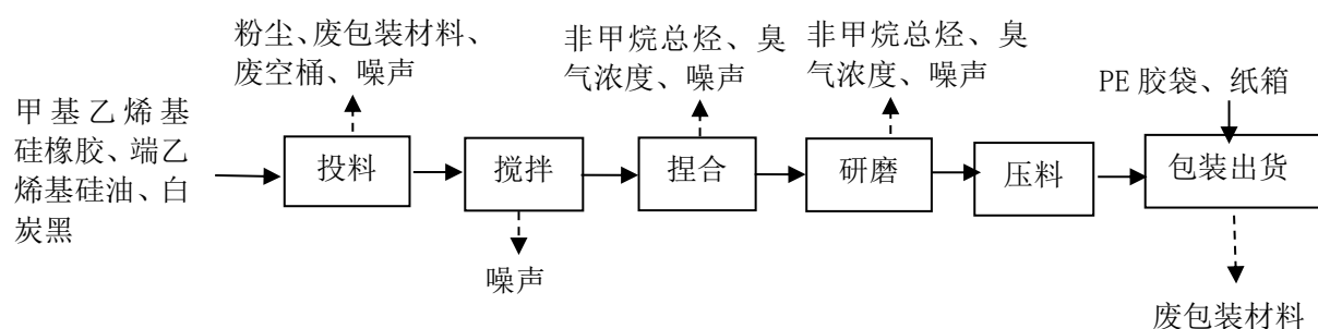
图 2-3 项目硅胶生产工艺流程图
