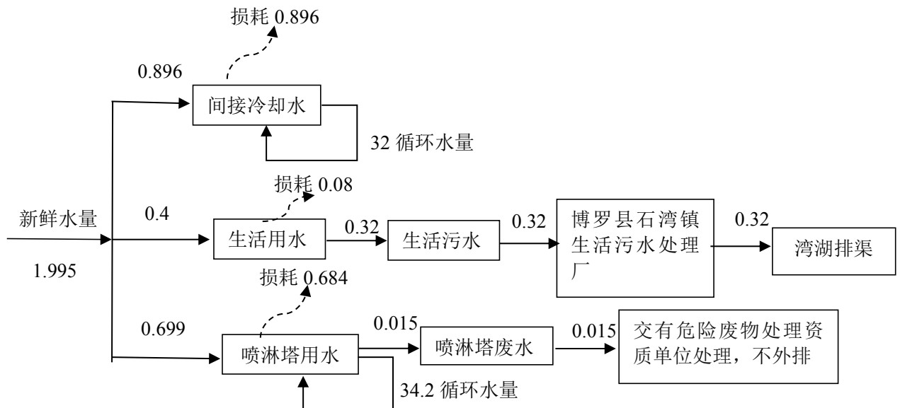
图 2-1 项目水平衡图 (m³/d)
