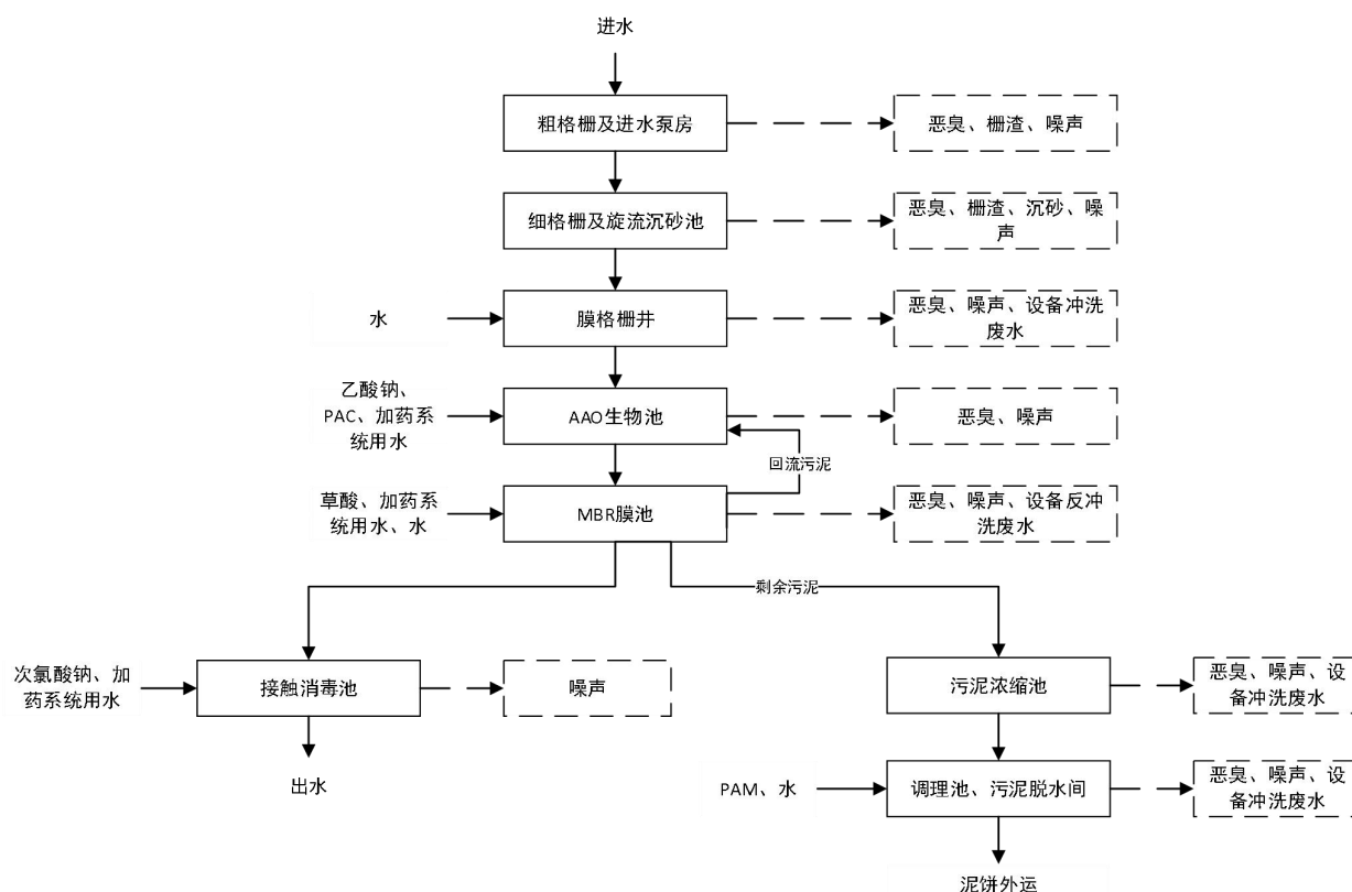
图 4 营运期工艺流程图及产污环节图
