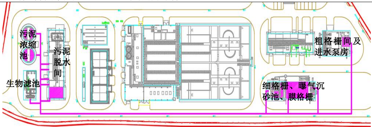
项目废气密闭罩和集气管道收集图
