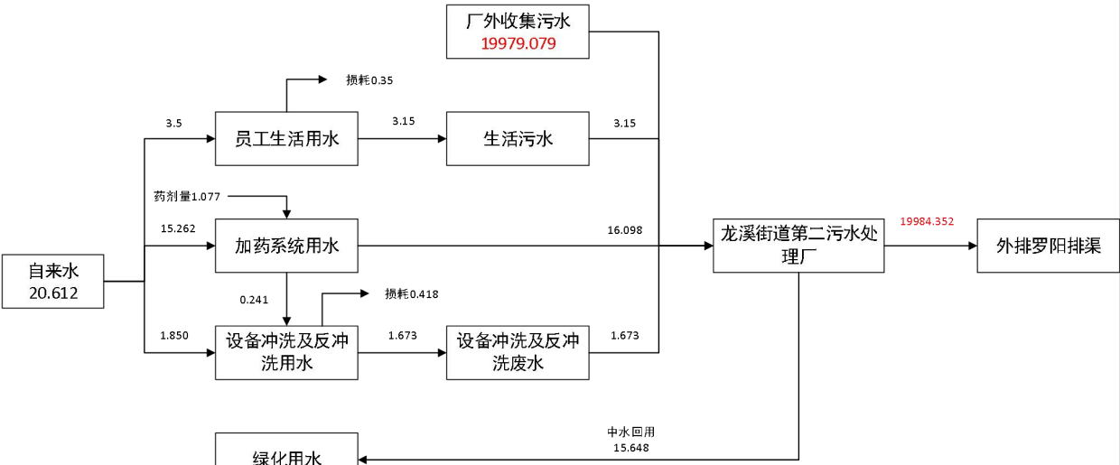
图 1 项目水平衡图-晴天 (t/d)
