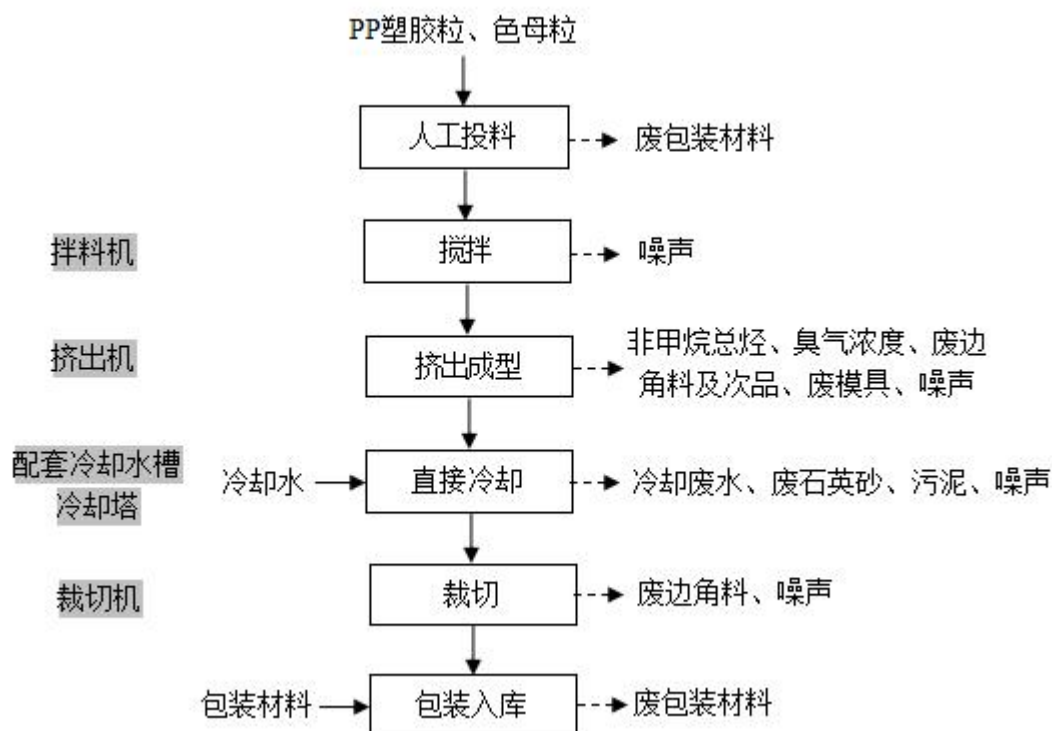
图 2-3 项目 PP 塑料管生产工艺流程及产污环节图
