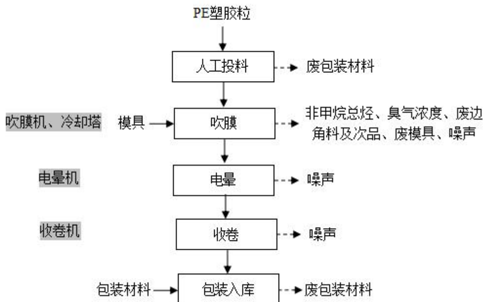
图 2-2 项目 PE 保护膜生产工艺流程图
