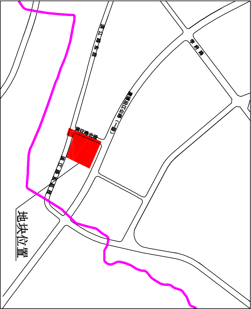
附图1：区位图
