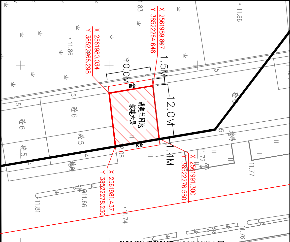
附图：总平面图
