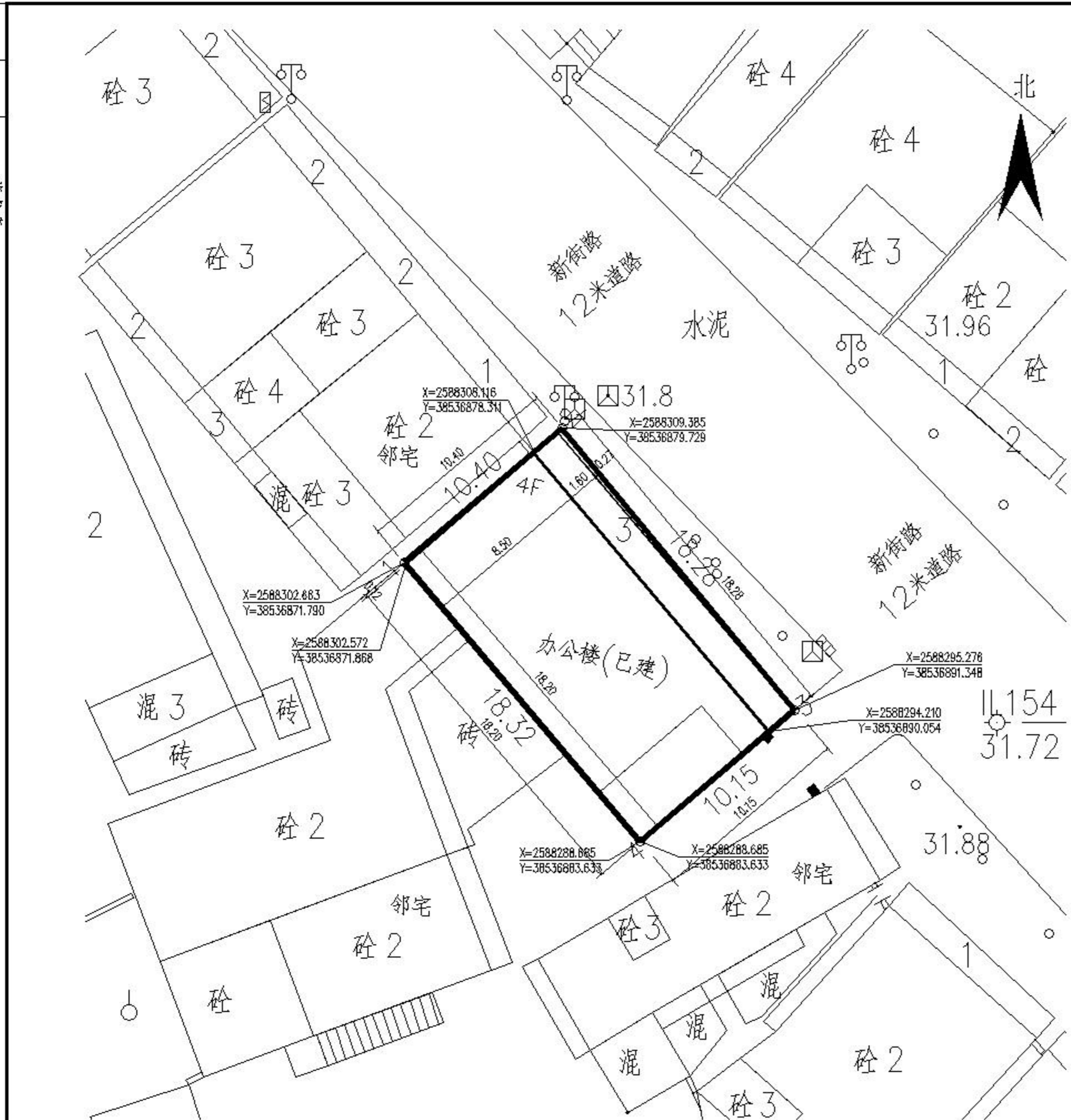
总平面图 1:150
