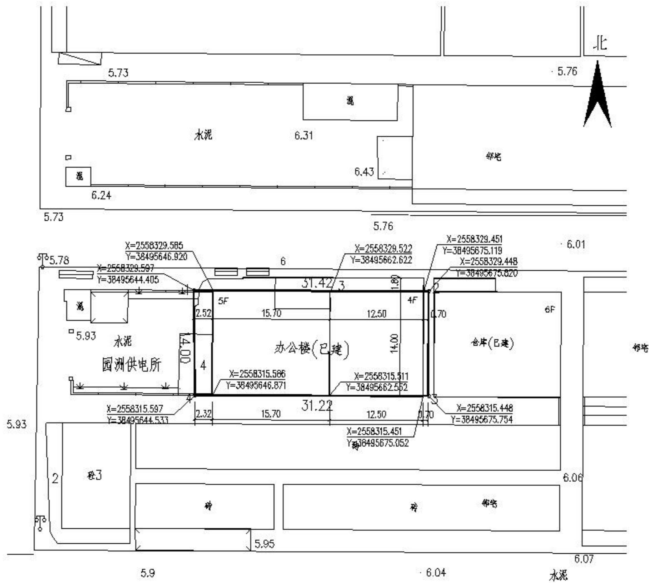
总平面图 1:300
