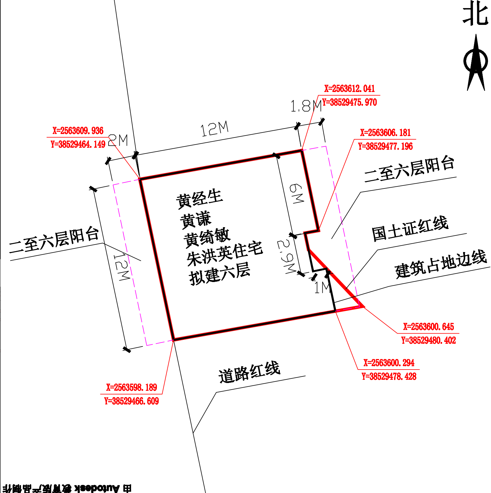
附图二：总平面图
