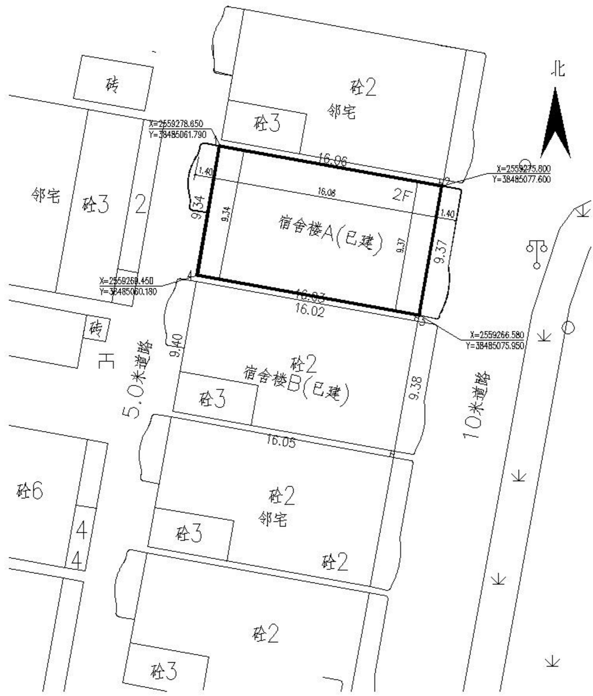
总平面图 1:150
