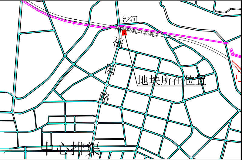
图例
