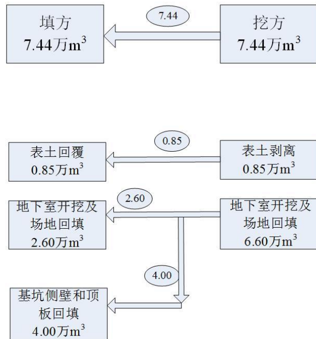
图 3.7-1 土石方平衡框图
